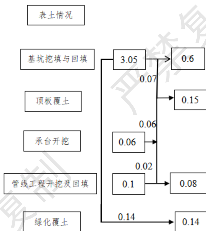
图 1.3-1 土石方流向框图 单位: 万 m 3
