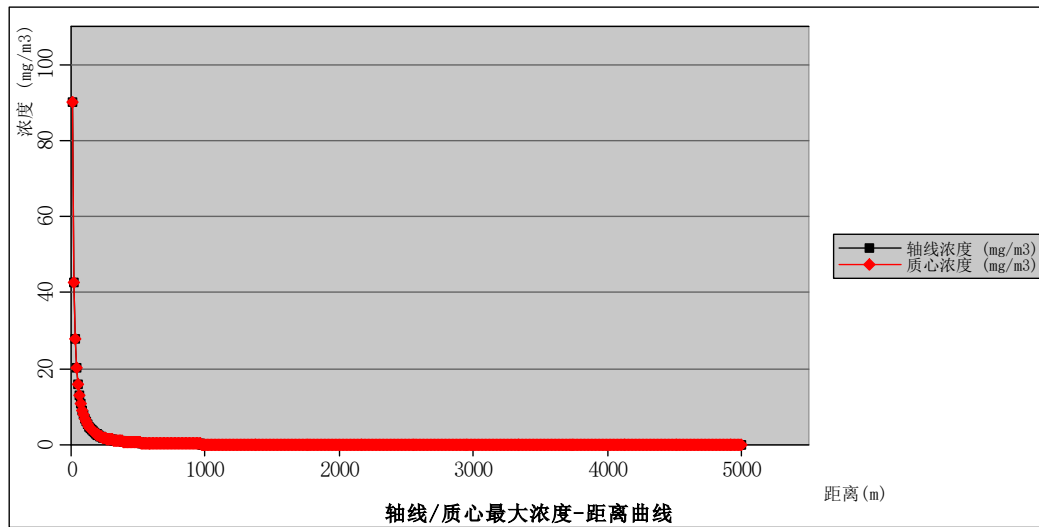
图 6.6-7 液氨泄漏轴线/质心最大浓度图（最常见气象条件下）
