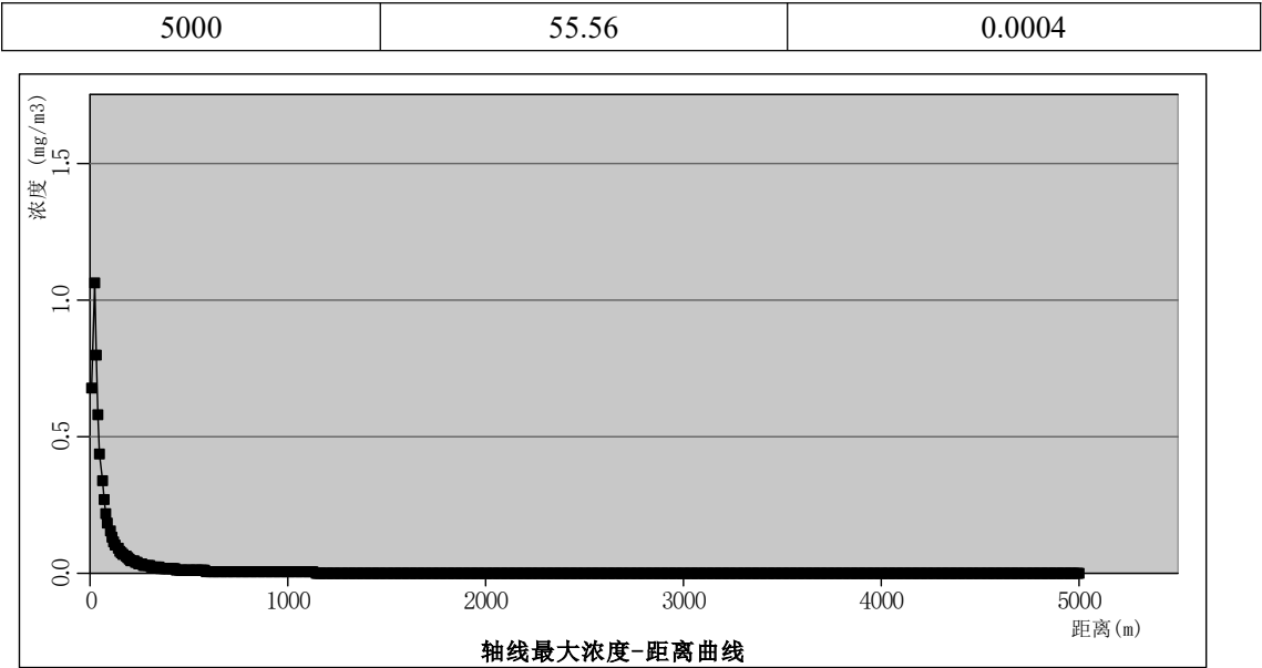
图 6.6-1 硫酸泄漏轴线/质心最大浓度图（最不利气象条件下）
