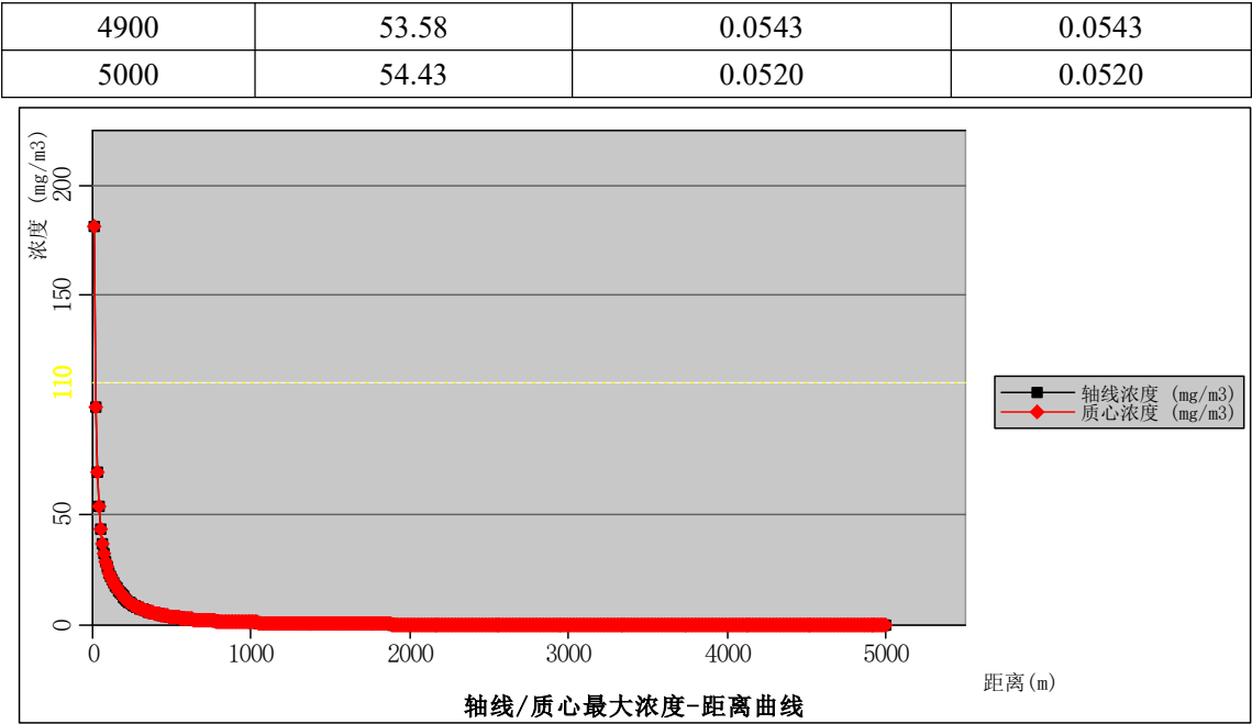
图 6.6-5 液氨泄漏轴线/质心最大浓度图（最不利气象条件下）
