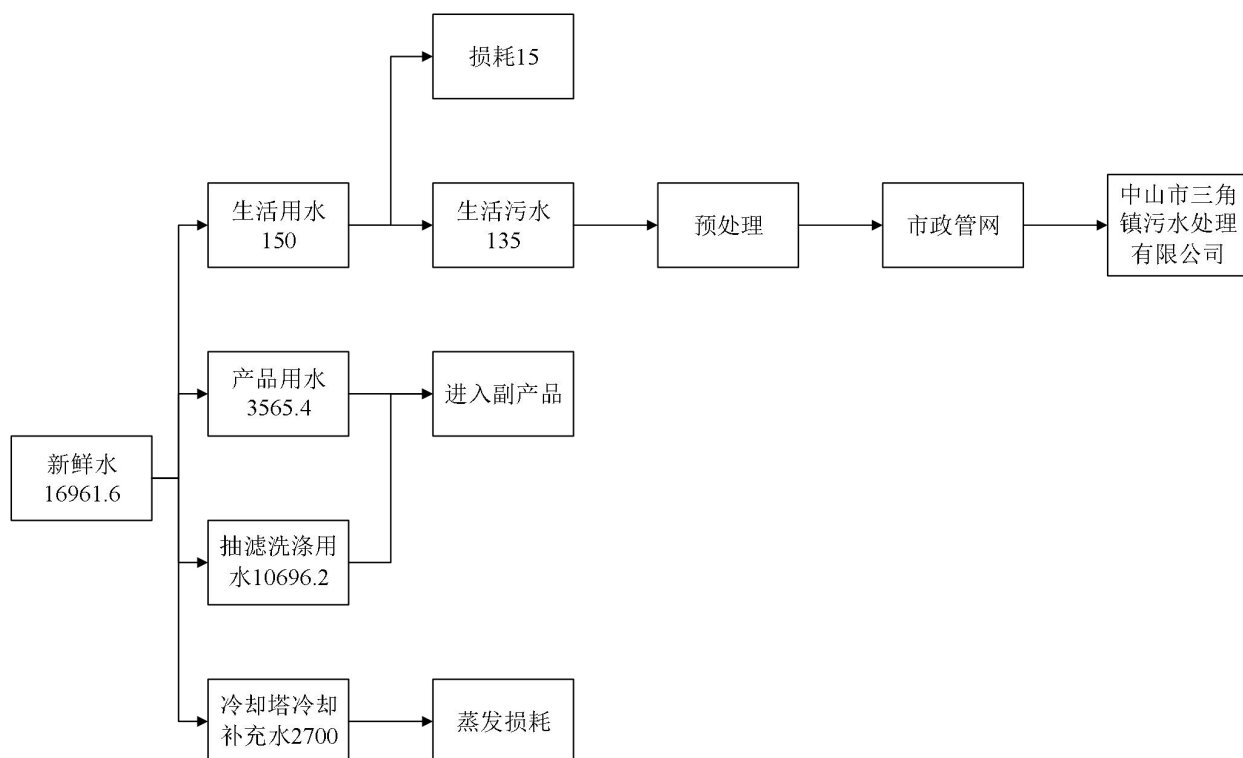
图 4.2-2 年水平衡图 (t/a)
